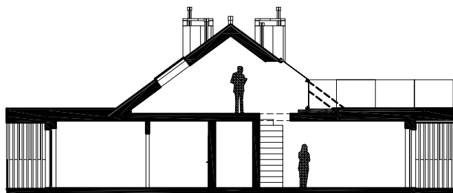
PRZEKRÓJ
